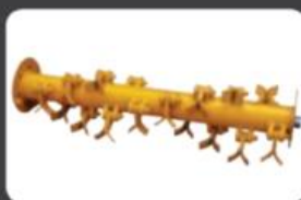
System spiralnego rozmieszczenia noży w dwóch rzędach „OVERLAP”
